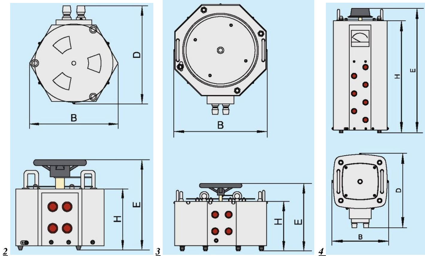
Autotransformatoare dimensiuni :
